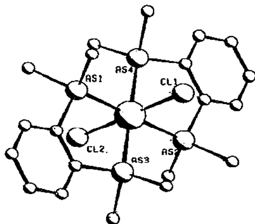
Fig. 12. tr - [\text{Tc}(\text{diars})_2\text{Cl}_2]^+ .
