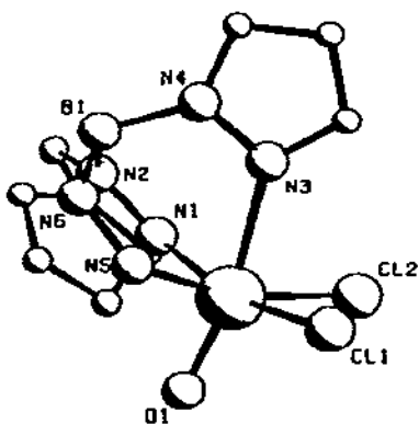
Fig. 24. Tc(HBPz 3 )Cl 2 O.
