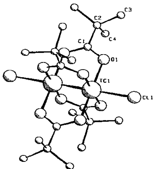
Fig. 28. \text{Tc}_2\text{Cl}_2(\text{OOCCMe}_3)_4 .
